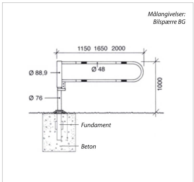
BG beskytter ved udkørsel, når et sæt er opstillet forskudt på en gang- og cykelsti
